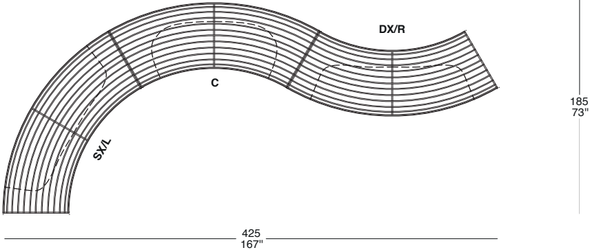
SOP 09 SX
